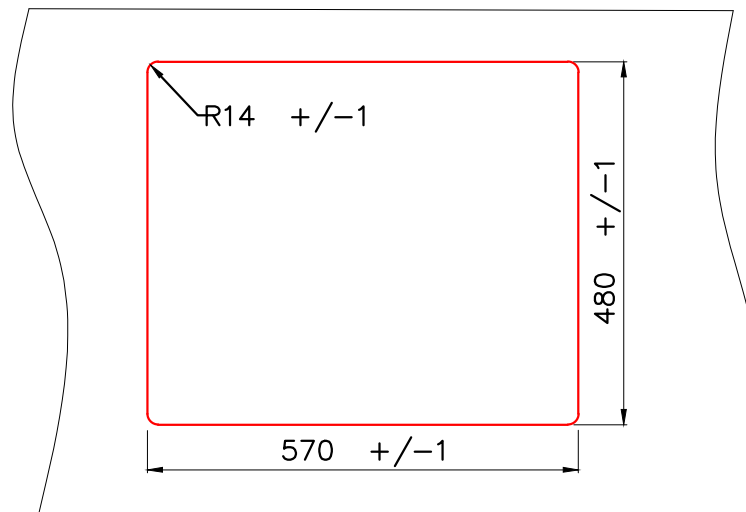
Врезной монтаж мойки (I)
