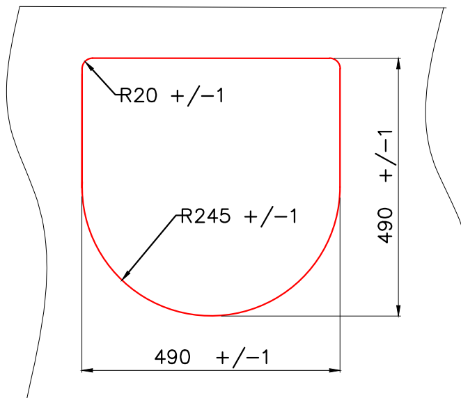
Врезной монтаж мойки (I)
